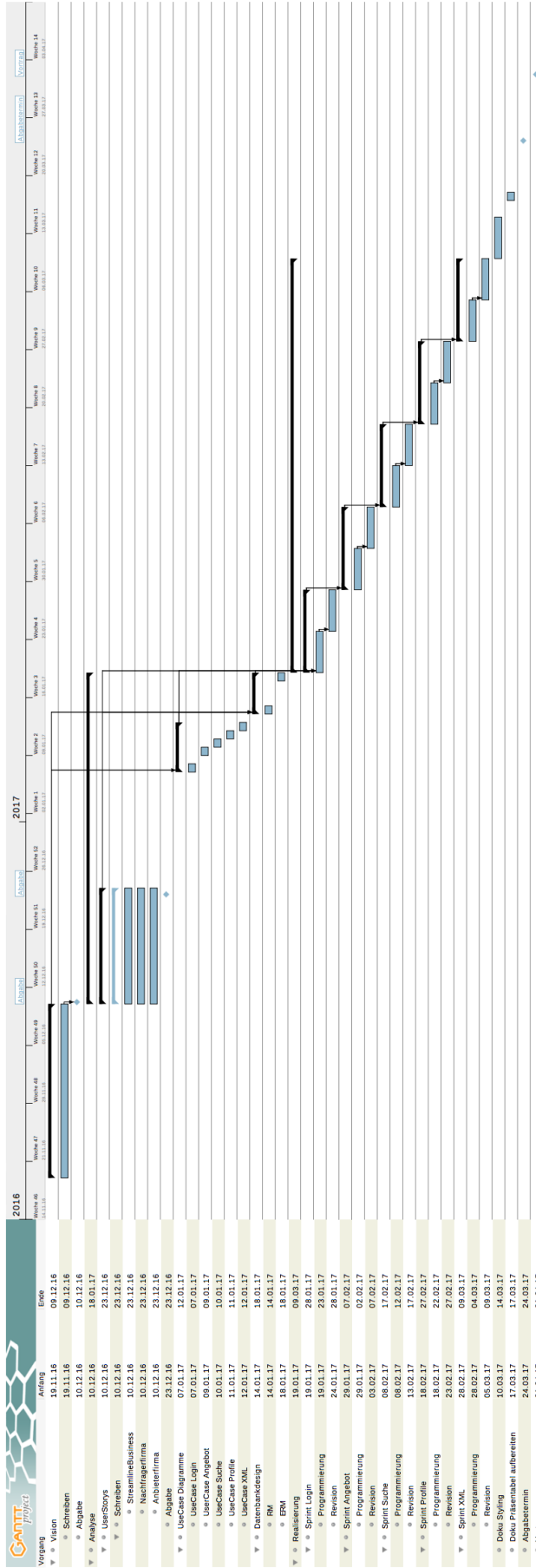
Abbildung 13: Zeitplanung
