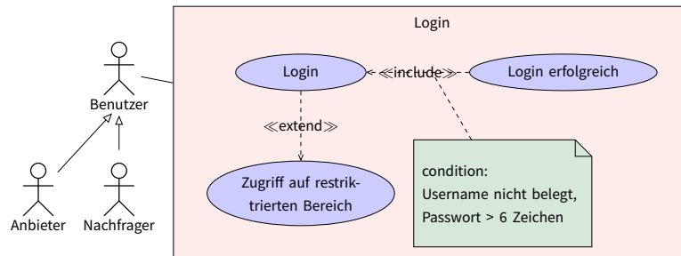
Abbildung 4: Login vorgang
